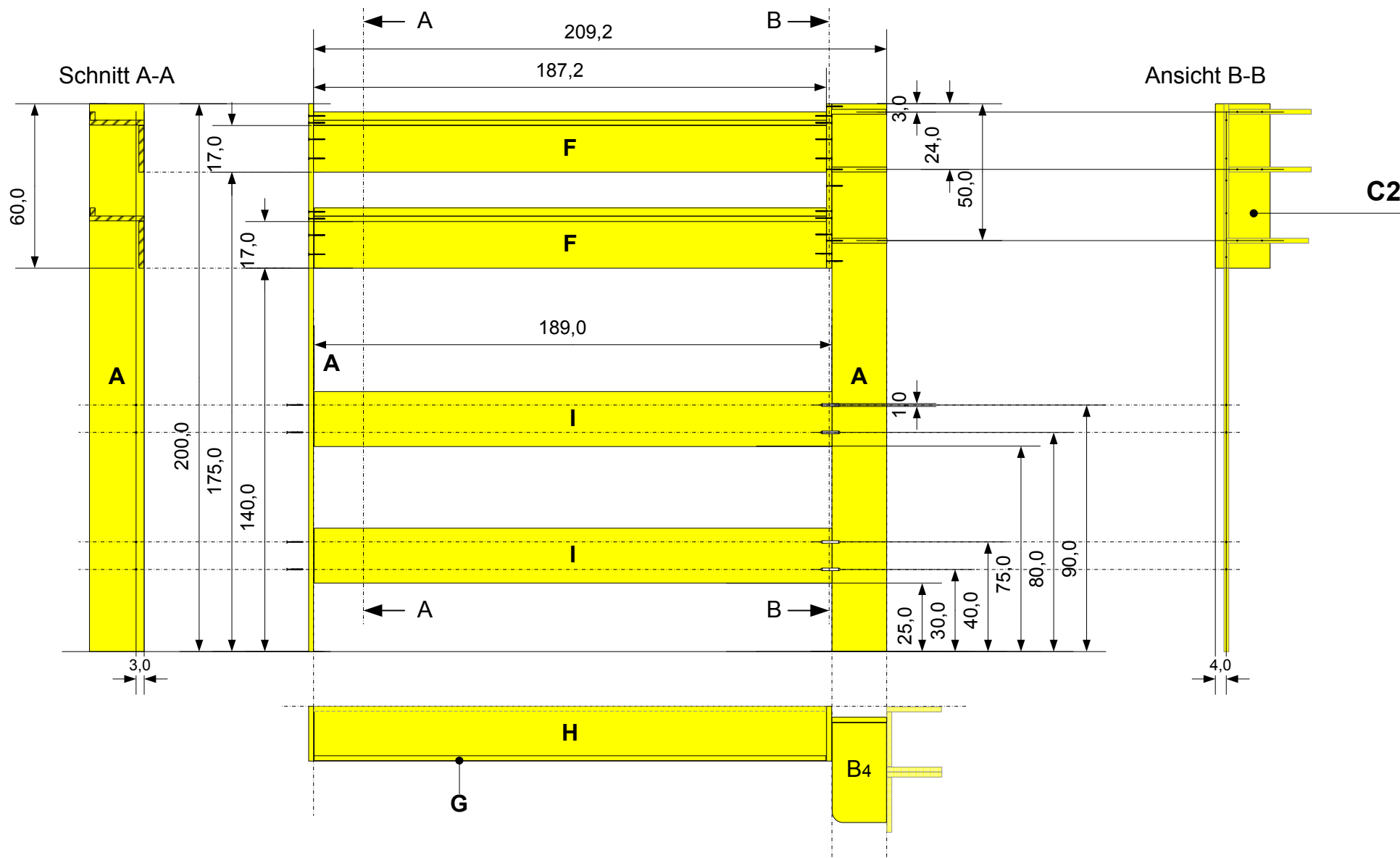
Liegesofa (etwa 80/140 x 200 - Beddinge, IKEA) mit Umbau , Bettkasten, Wäschebox-Regal und Seitenregal Aufriß pm – 2011-01-10 - M 1 : 20 - Maße: cm
